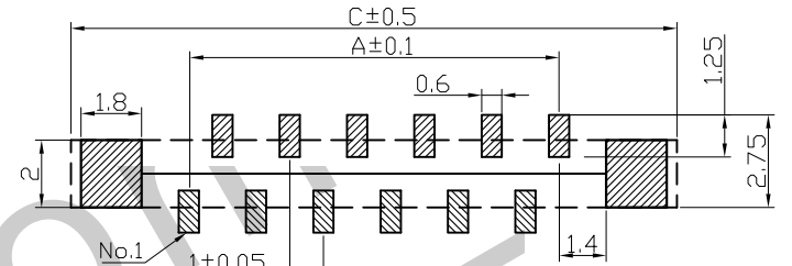
适用线路板 RECOMMENDED PCB LAYOUT
