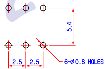
P.C.B DIAGRAM
