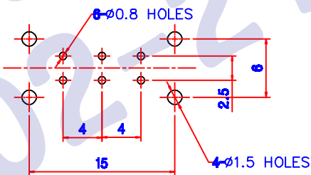
P.C.B DIAGRAM
