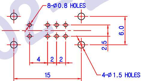
P.C.B DIAGRAM
