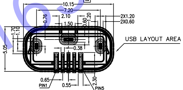
RECOMMEND PCB LAYOUT PCB图仅供参考
