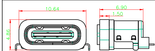
加防水圈示意图
