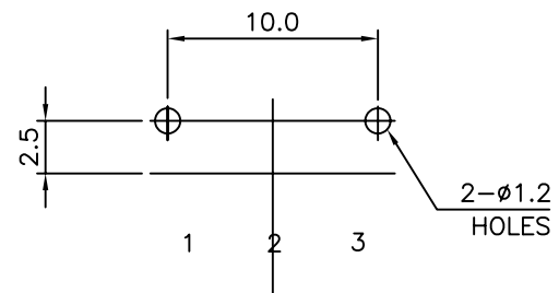
P.C.B POSITION
